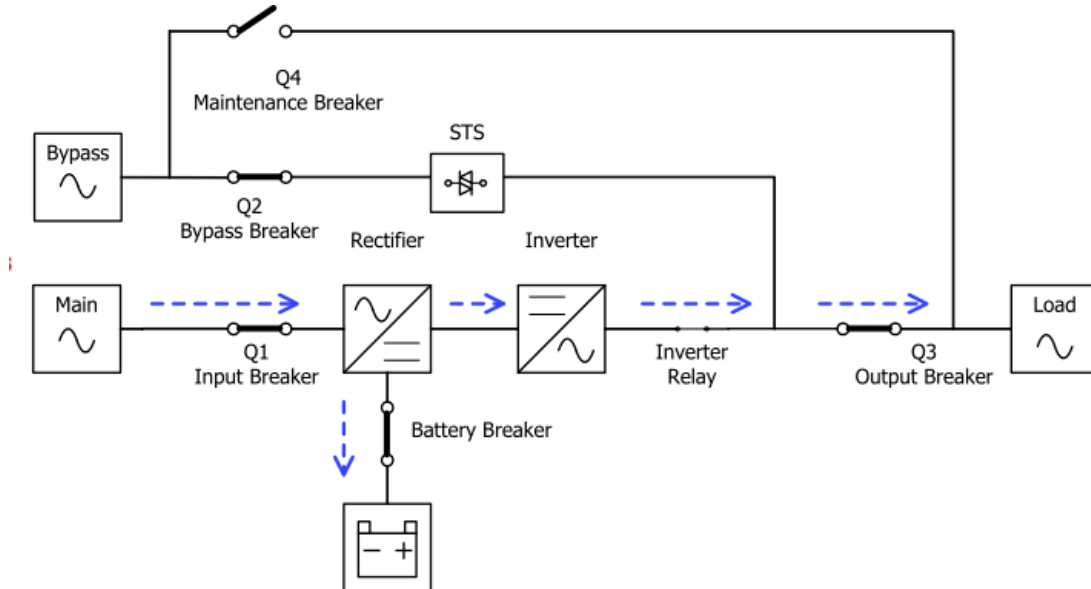
Figura 4.3 - Diagrama de operación en modo line
