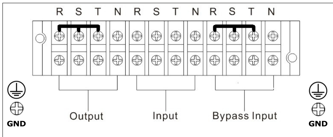
Figura 6.3 - Bloque de terminales
