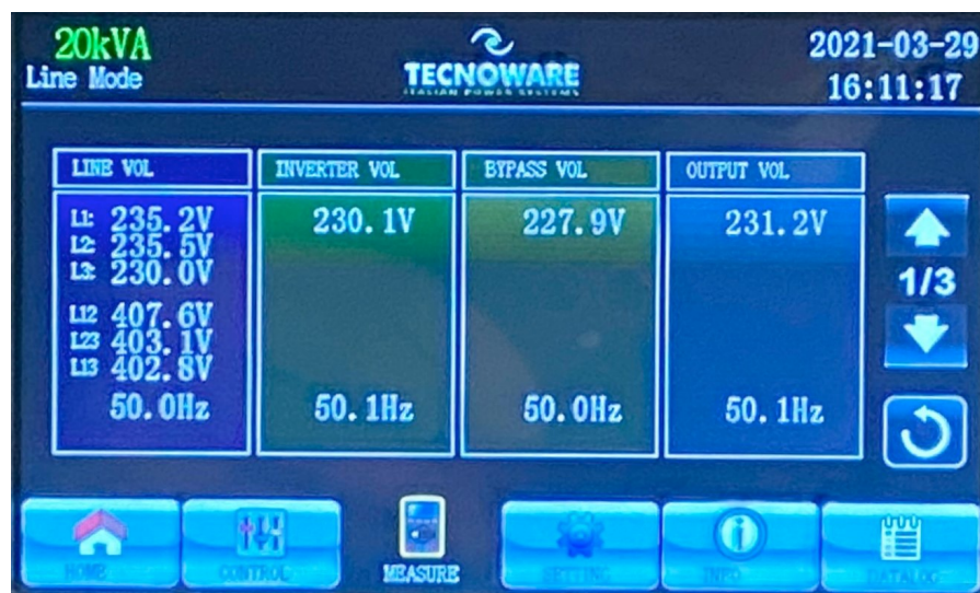
Figura 5.16 - Pantalla MEDIDAS página 1
