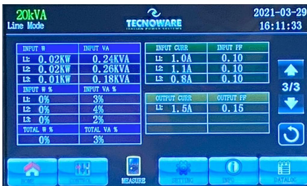
Figura 5.18 - Pantalla MEDIDAS página 3
