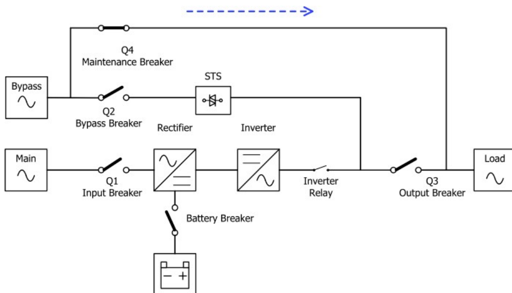
Figura 4.8 - Diagrama de funcionamiento del modo Bypass de mantenimiento
