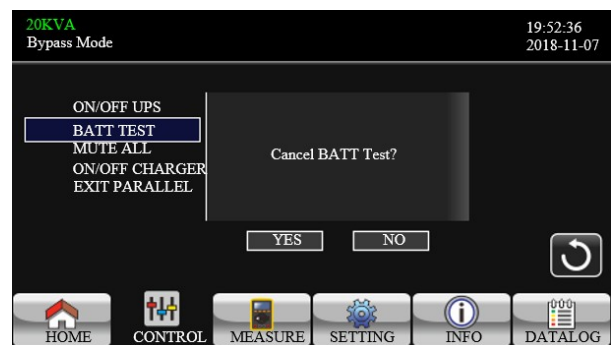
Figura 5.10 - Cancelación del Test de baterías
