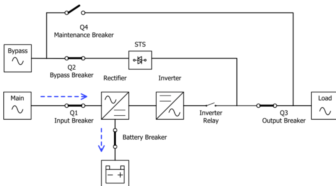
Figura 4.2 - Diagrama de funcionamiento en modo Stand-By
