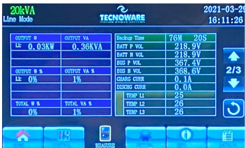
Figura 5.17 - Pantalla MEDIDAS página 2
