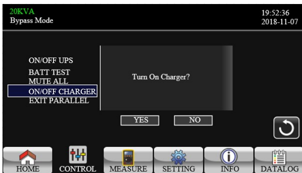
Figura 5.13 - Encienda el Cargador de batería
