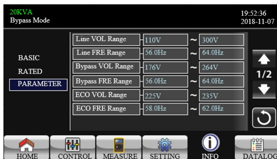
Figura 5.25 - Pantalla de información de PARÁMETROS página 1
