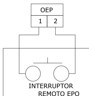
Figura 6.4 - EPO (apagado de emergencia)
