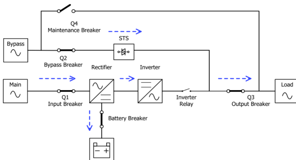
Figura 4.6 - Diagrama de funcionamiento del modo ECO
