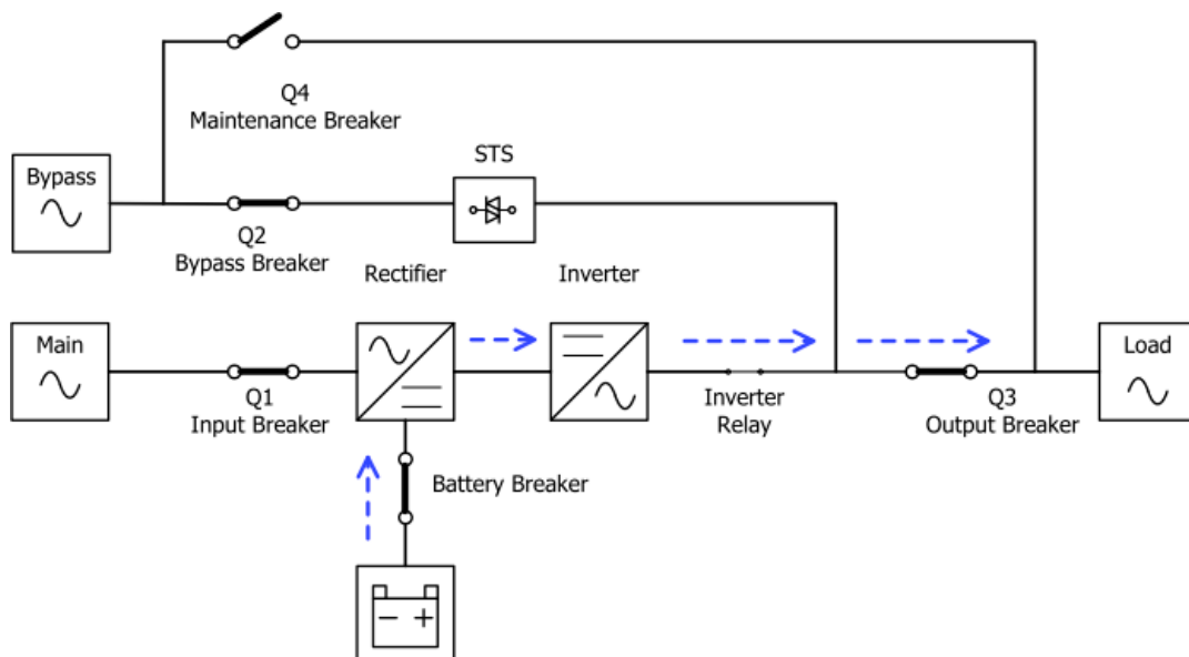
Figura 4.4 - Diagrama de funcionamiento en modo batería
