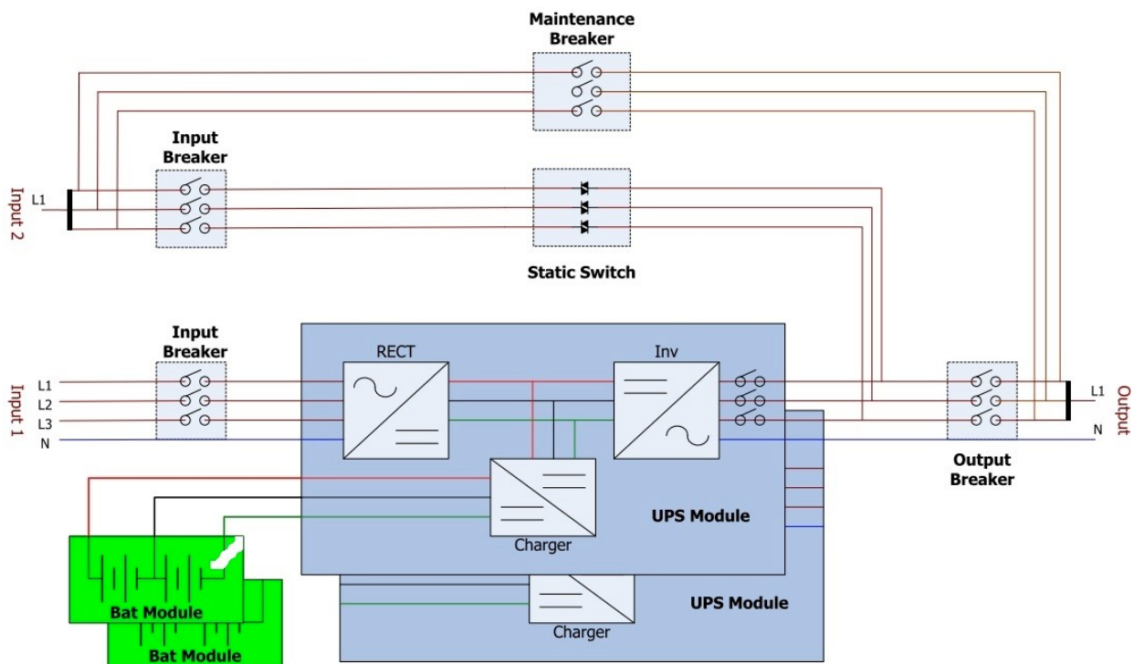
Figura 4.1 - Diagrama de bloques y conexiones
