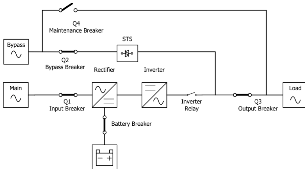
Figura 4.7 - Diagrama de operación del modo OFF
