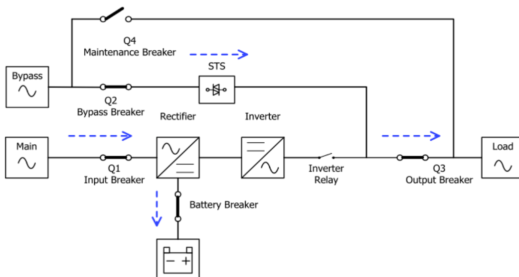
Figura 4.5 - Diagrama de funcionamiento del modo bypass
